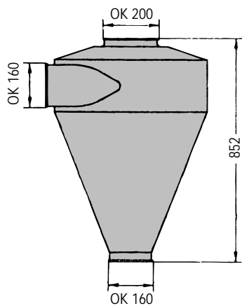
RC サイクロン, ガルバナイズ (ダストサイクロン) 131 000 047
