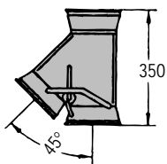
2又切替管45°, グレー 122 000 692
