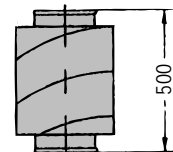
0.5m サイレンサー, ガルバナイズ 125 500 544
