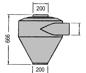
ICサイクロン 30°, グレー (交換可能フィルター付) 121 000 719
