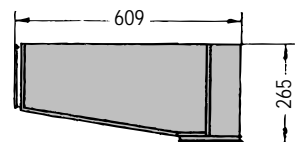
排出ヘッド, ガルバナイズ 122 000 688
