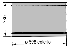
延長ホッパー, ブルー 122 000 013
