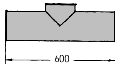
分岐管90°, グレー OK 160/100/160 122 000 461
