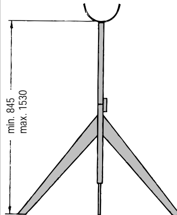
高さ調整可能パイプサポート, グレー 122 000 705
