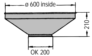
ホッパー (ガード無), ブルー 122 050 051
