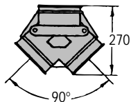
2又切替管90°, グレー 124 000 014
