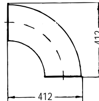
90° ベンド, ガルバナイズ R = 300 122 050 116
