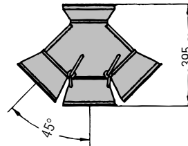
3又切替管 45°, グレー 122 050 131
