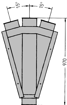
3又切替管15°, グレー 122 000 682
