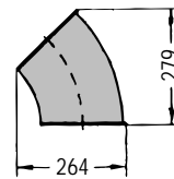
45° ベンド, ガルバナイズ R = 300 122 050 115
