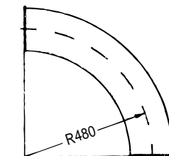
90° ベンド, ガルバナイズ 122 020 124
