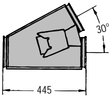
2又切替管30°, グレー 122 000 690
