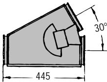
2又切替管30°, グレー エアシリンダー取付用 シリンダー含まず 122 000 697
