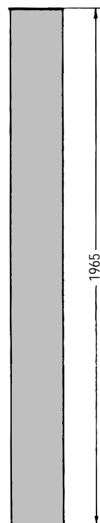
2.0m パイプ, ガルバナイズ 122 050 083
