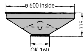
ホッパー(ガード付), ブルー 121 100 135
