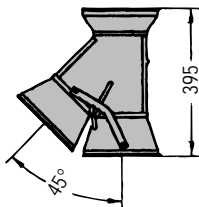
2又切替管 45°, グレー 122 050 130
