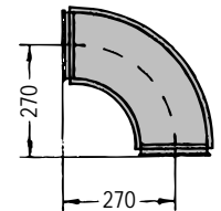
90° ベンド, グレー R = 240 (排気/通風用). 板厚: 1.0 mm 122 020 094
