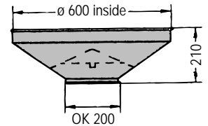
ホッパー(ガード付), ブルー 121 106 071
