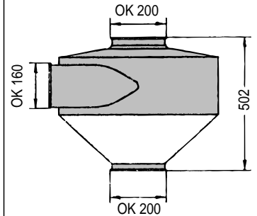
UCサイクロン, グレー (排気用サイクロン 1xクイックリリース・クランプ付) 122 000 687
