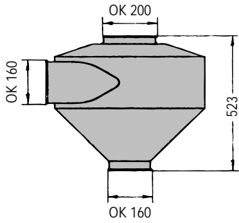
UC サイクロン, ガルバナイズ (排気用サイクロン) 122 000 698
