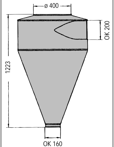
RCサイクロン, ブルー (ダストサイクロン) 131 020 099
