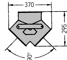
2又切替管 90°, グレー 122 050 006
