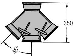
3又切替管45°, グレー 122 000 693
