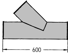
分岐管45°, グレー OK 160/100/160 122 000 323
