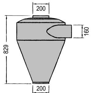
ICサイクロン 20°, グレー (交換可能フィルター付) 131 025 101
